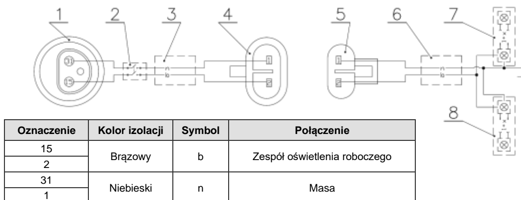
Rys. 54. Schemat instalacji elektrycznej oświetlenia roboczego
