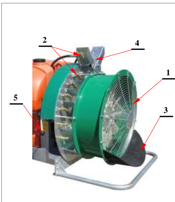
Rys. 31. Przystawka sadownicza D8
