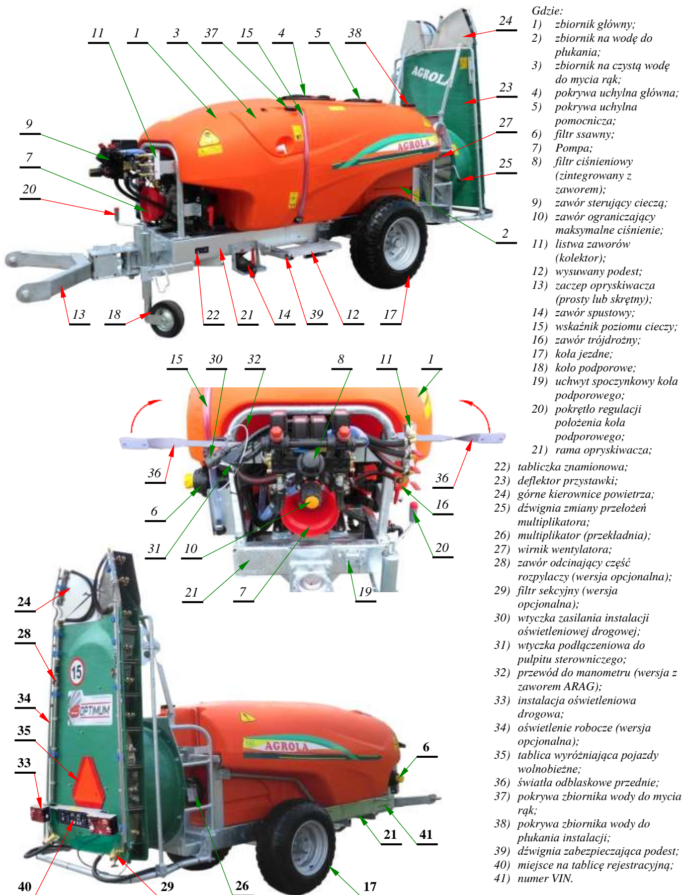
Rys. 5. Widok opryskiwacza sadowniczego przyczepianego z przystawką Optimum
