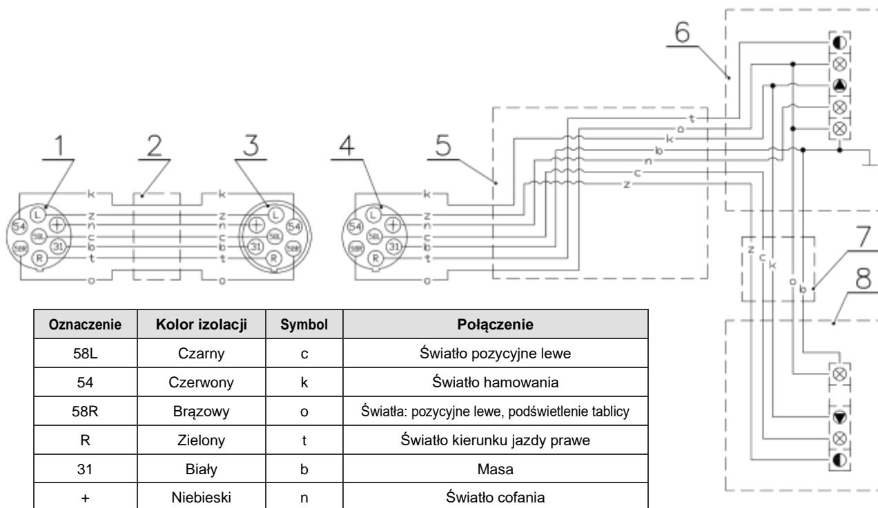
Rys. 53. Schemat instalacji elektrycznej oświetlenia drogowego
