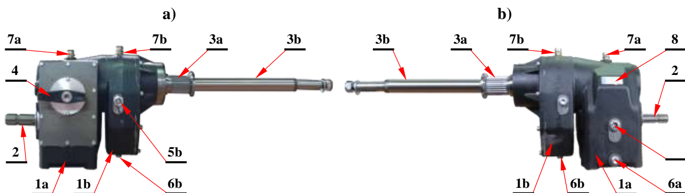
Rys. 50. Multiplikator (przekładnia) z inwerterem MSC-C
