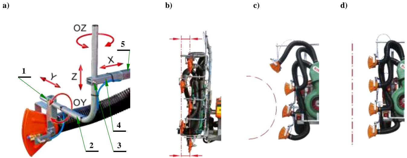
Rys. 41. Regulacja i ustawienie dyfuzorów w przystawkach Ribes
