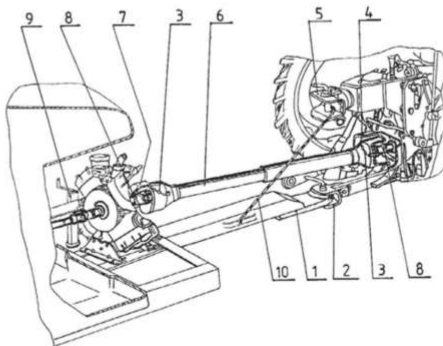
Rys. 68. Agregowanie opryskiwacza z ciągnikiem
