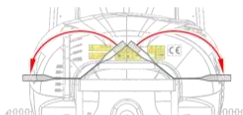
Rys. 60. Ustawienie przedniej instalacji świateł odblaskowych w pozycji na czas przejazdów drogowych
