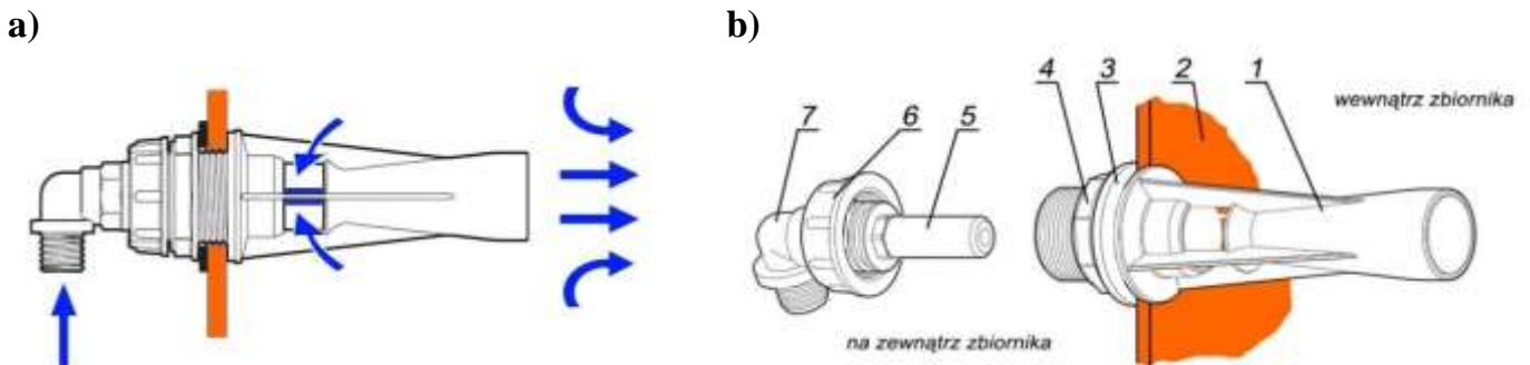
Rys. 16. Mieszadło hydrauliczne:
