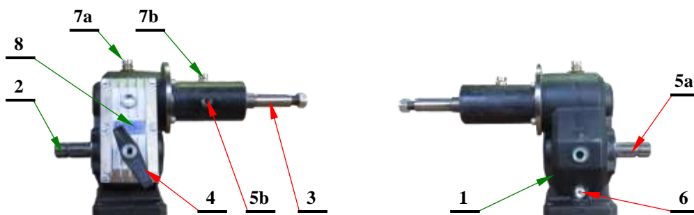
Rys. 46. Multiplikator (przekładnia) M47CS
