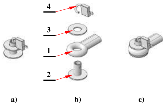
Rys. 66. Zabezpieczenie antykradzieżowe montowane na dyszlu prostym -D2PR-A1.00.00
