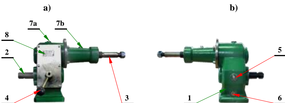
Rys. 47. Multiplikator (przekładnia) TM35
