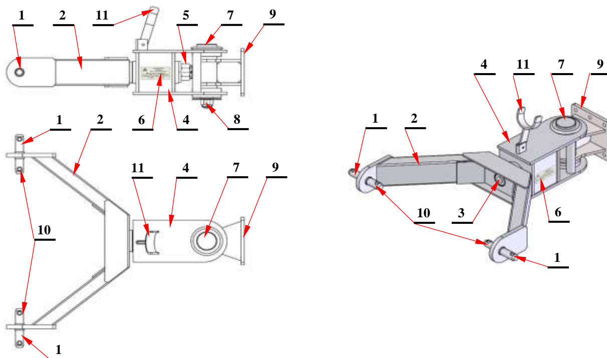
Rys. 64. Schemat zaczepu skrętnego kategorii 2N (kategoria 2 zwężona)
