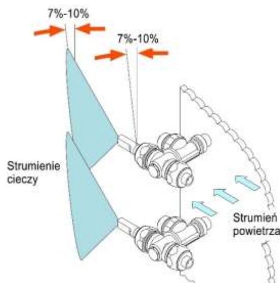
Rys. 44. Schemat montażu rozpylaczy płaskostrumieniowych
