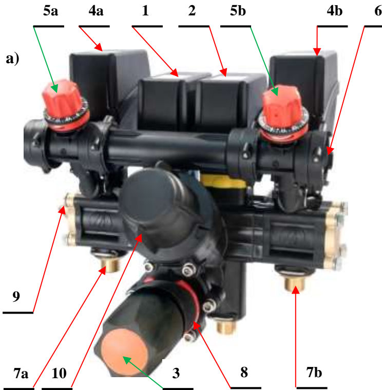
Rys. 21. Elektrozawór ARAG sterujący cieczą do współpracy z manualnym pulpitem sterującym:
