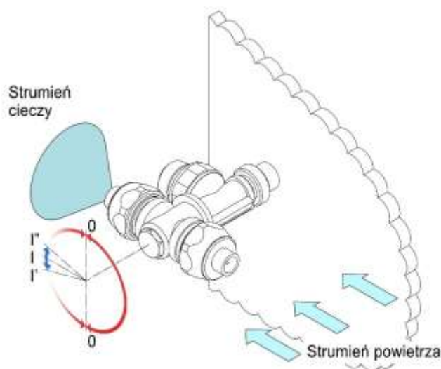
Rys. 43. Schemat nastawień korpusów rozpylaczy
