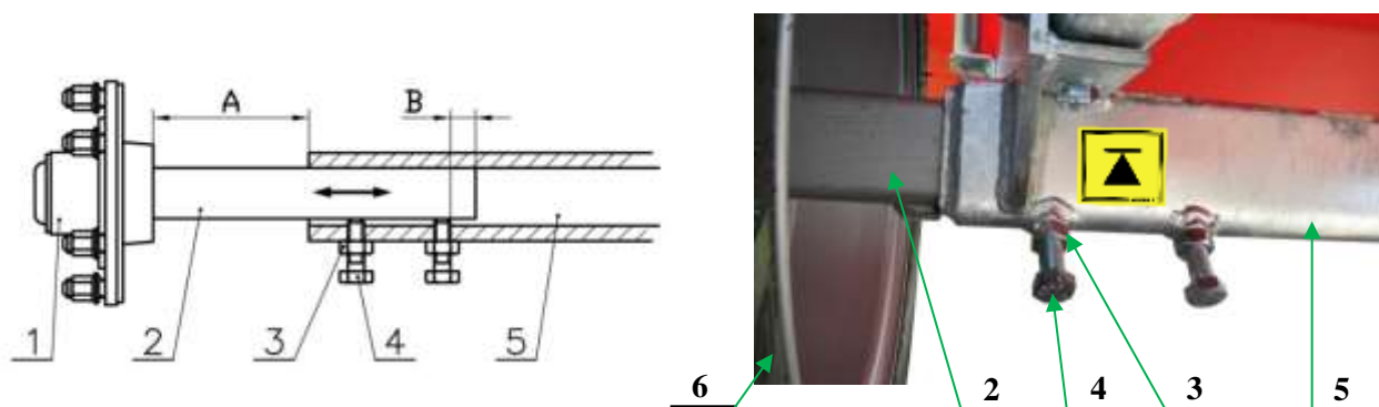
Rys. 52. Schemat regulacji rozstawu kół opryskiwacza
