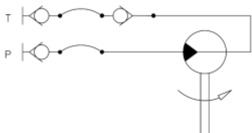
Rys. 57. Schemat hydrauliczny podłączenie silnika hydraulicznego pompy wirowej mieszadeł.
