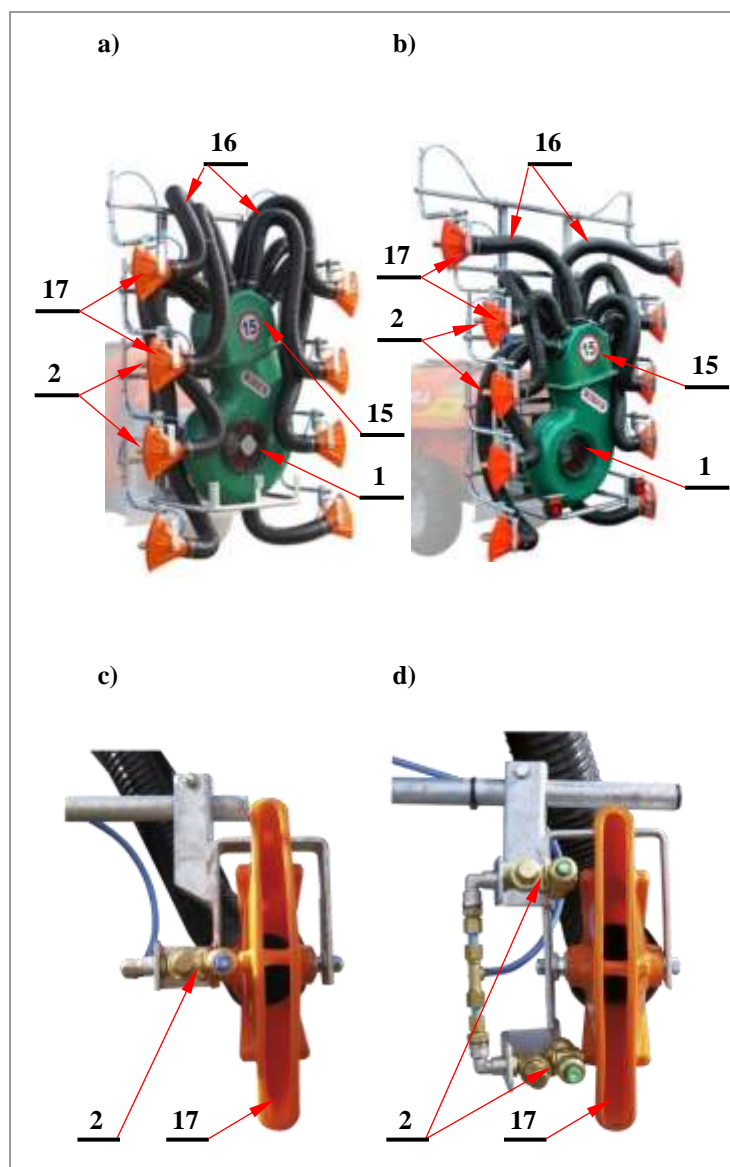
Rys. 40. Przystawka sadownicza Ribes
