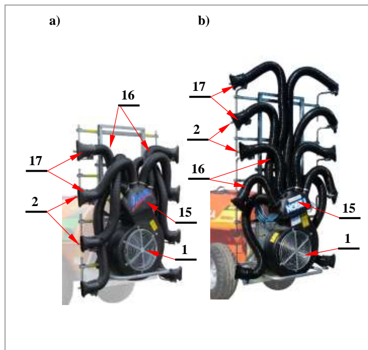
Rys. 39. Przystawka sadownicza Oktopus
