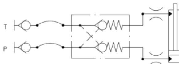
Rys. 58. Schemat hydrauliczny podłączenie cylindra hydraulicznego kierownic powietrza.
