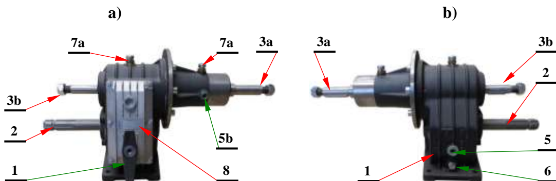
Rys. 49. Multiplikator (przekładnia) BIMA M60
