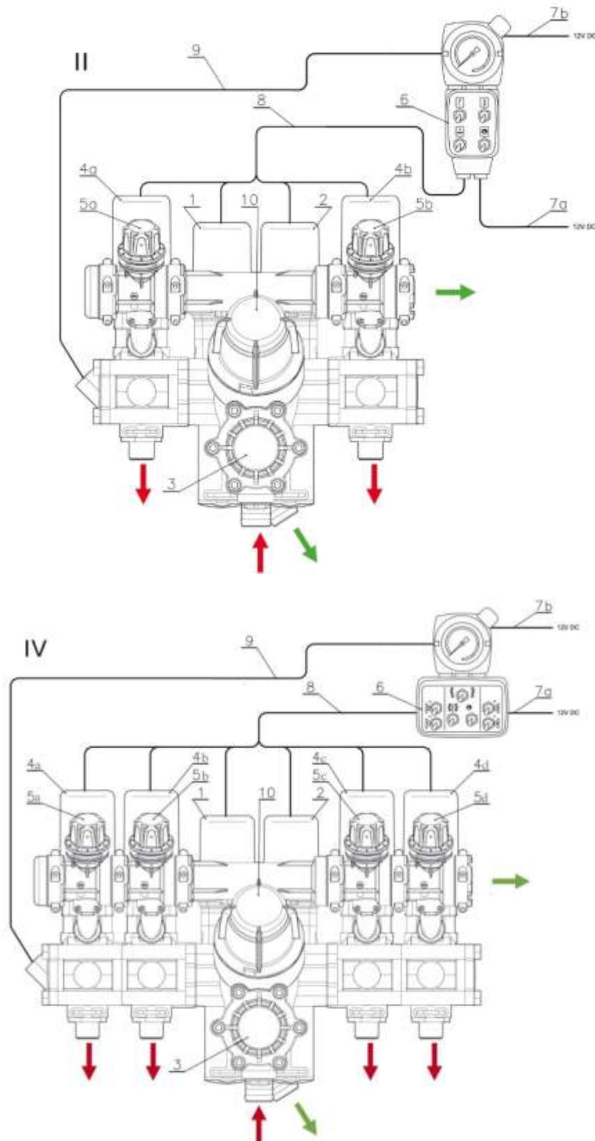
Rys. 22. Schematy elektrozaworów Arag
