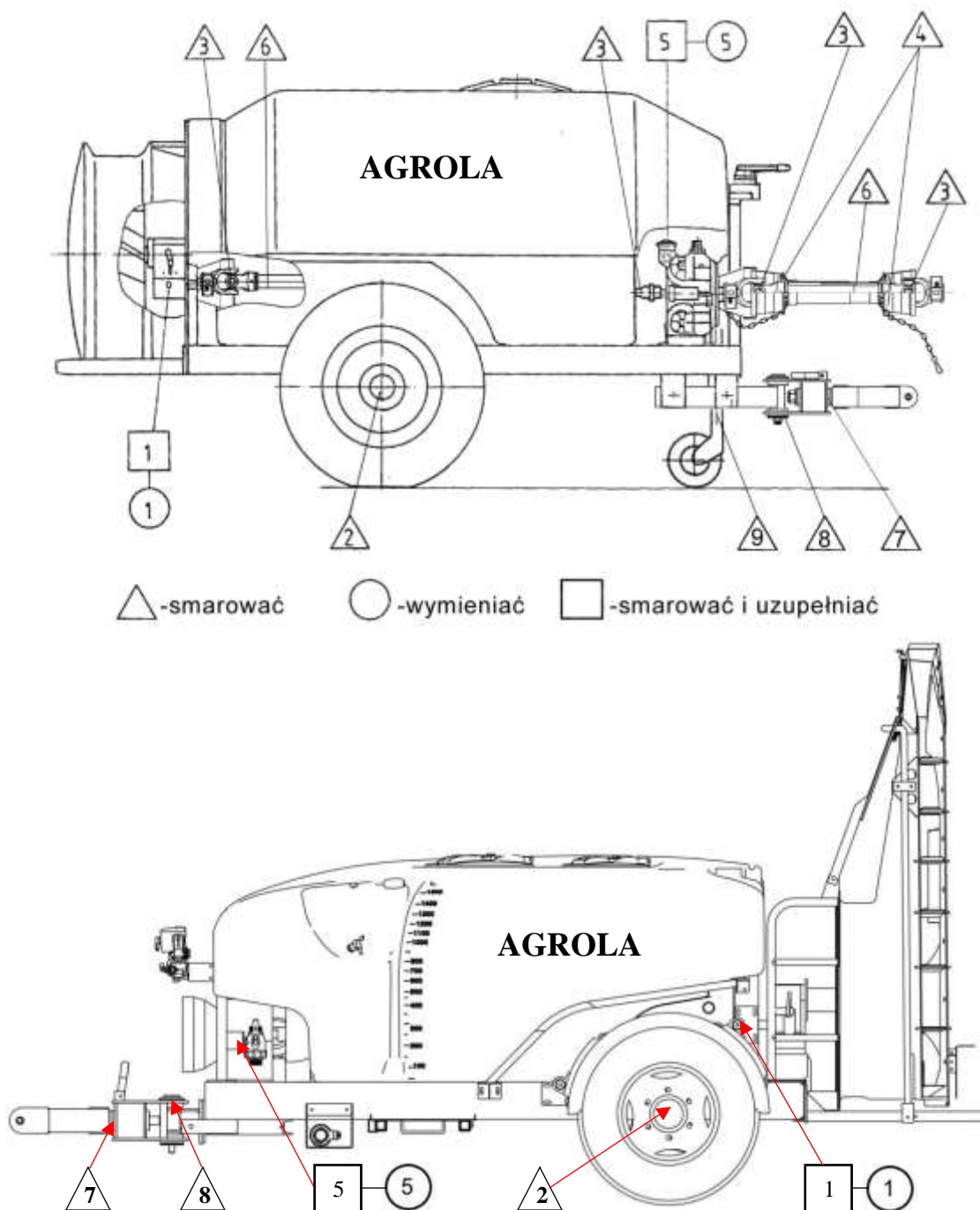
Rys. 69. Rozmieszczenie punktów smarowania
